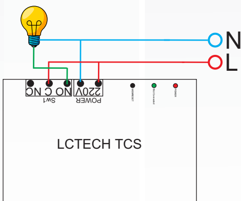
مدار اتصال
